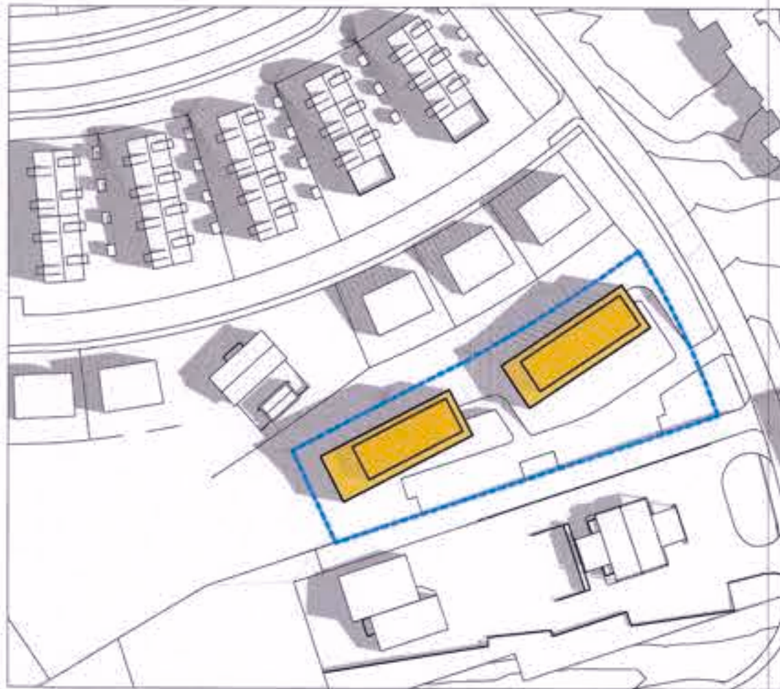
Sumarsólstöður KI: 9:00
