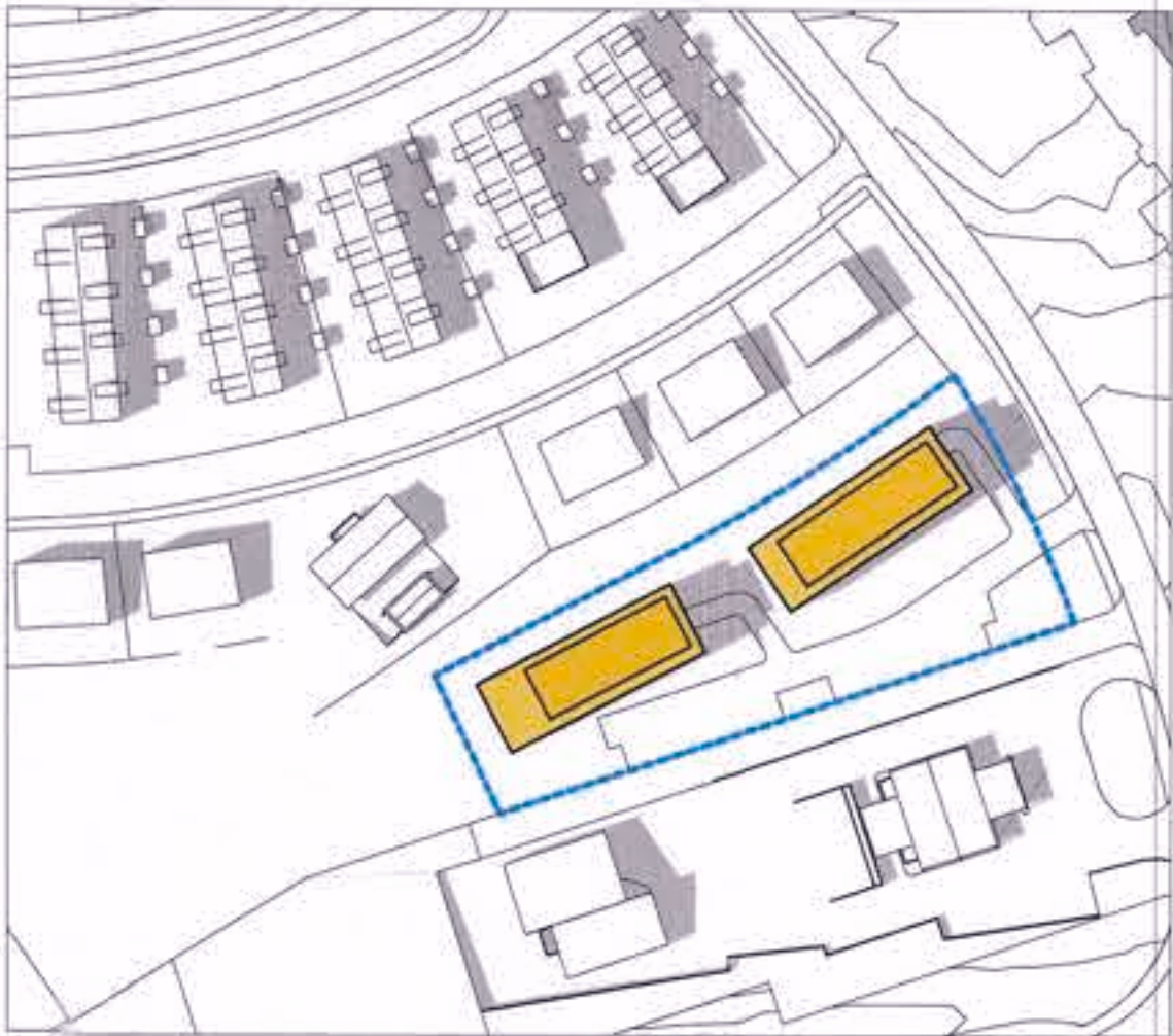
Sumarsólstöður KI: 17:00
